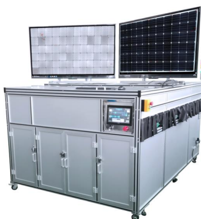
光伏组件 EL 和外观检测设备
