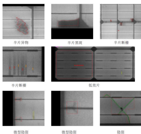
组件 EL 检测效果
