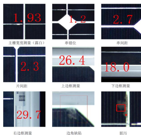
组件外观检测效果
